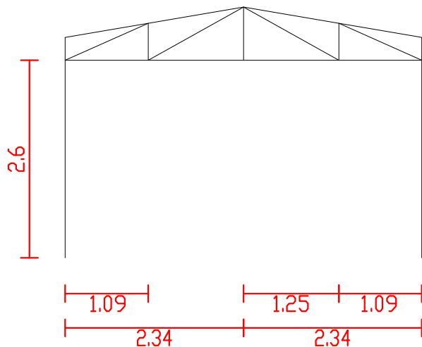
2D: FACHADA
