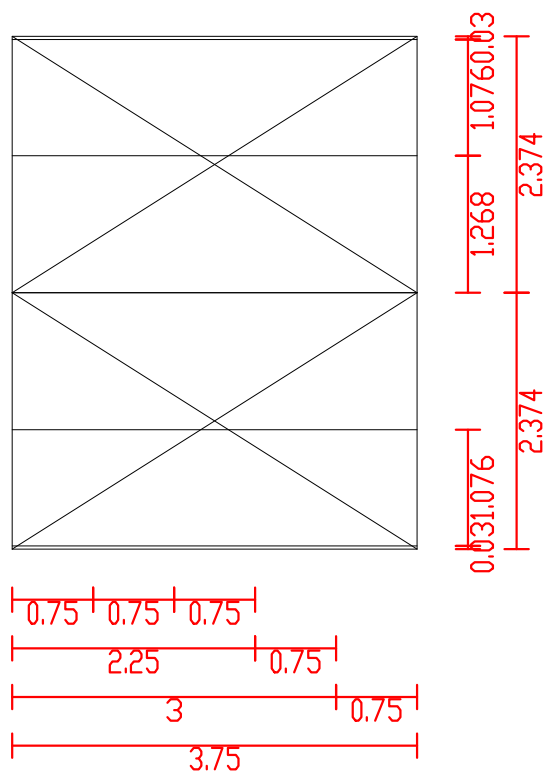
2D: COBERTURA
