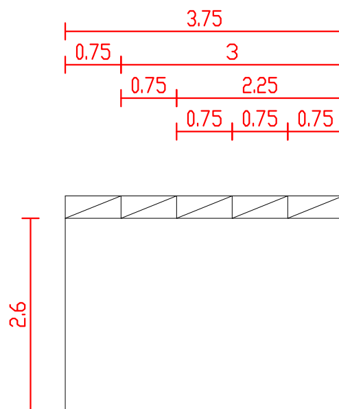
2D: VISTA LATERAL TRELIÇA
